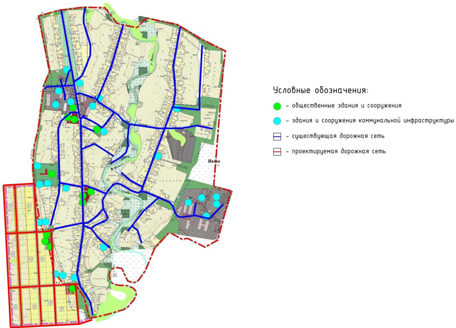
Рисунок 2. Существующая и проектируемая дорожные сети с. Миякитамак.
